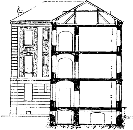
Budynek W Przekrój A-B
