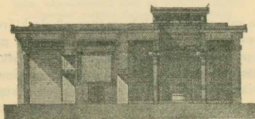
Fig. 11. Przekrój pionowy „mégaronu“ jednego z odrestaurowanych pałaców myceńskich pod. Perrot i Chipiez.
