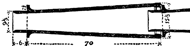
Fig. 3. Rury gliniane, służące do przeprowadzania wody i kanalizacji w pałacu w Knossos, pod. Thompson.
