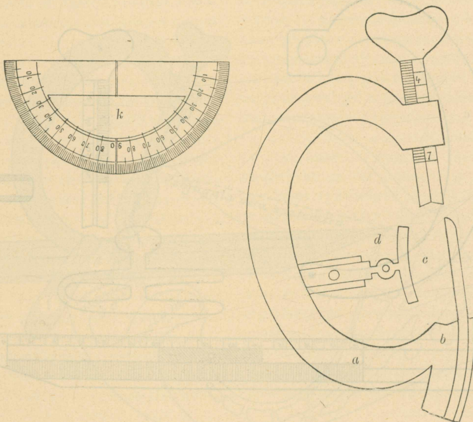
Fig. III. Przyrząd B.
