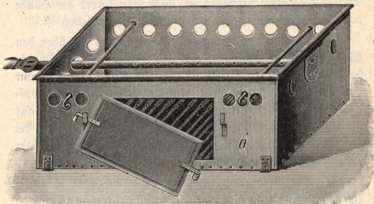
Fig. 17. Sterilisierapparat (Ofen).
